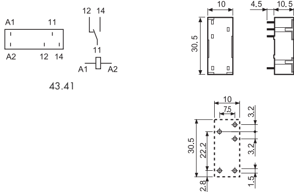
rysunek otworów montażowych
